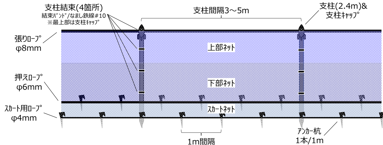
正面図 ※本体+スカート一体型の場合
